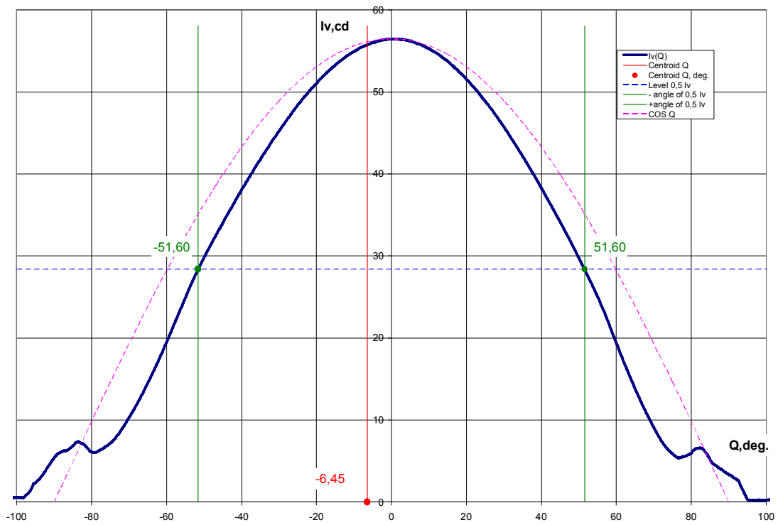
Диаграмма - Буферный фонарь красный
