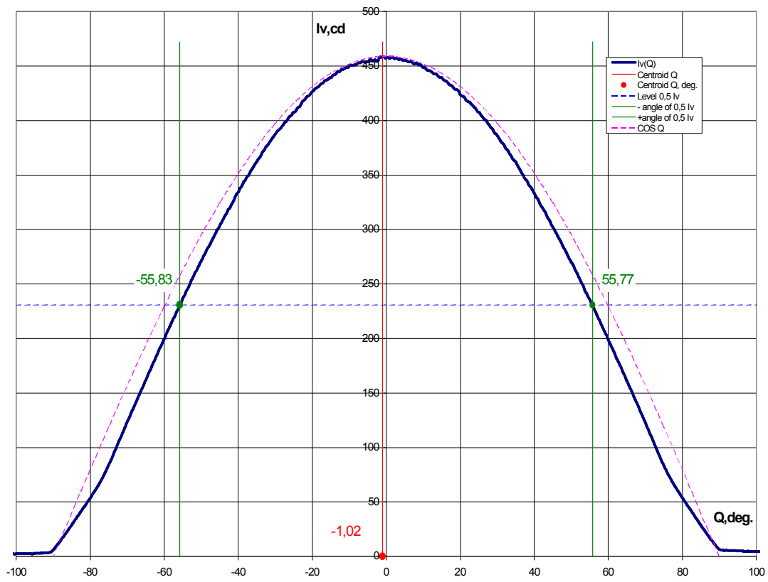
Диаграмма - Буферный фонарь белый
