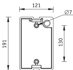
Установочные размеры
