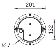
Установочные размеры
