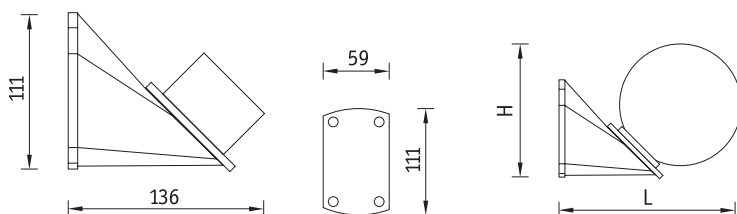
Установочные размеры
