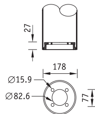
Установочные размеры
