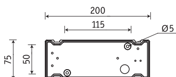
Установочные размеры
