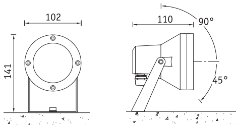
Установочные размеры
