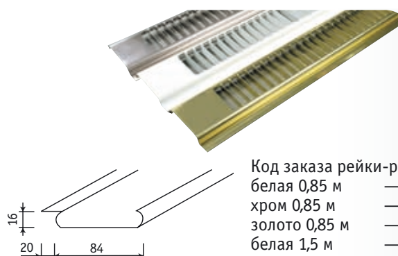
Схема рейки-решетки.
